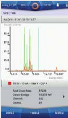
Spectra
